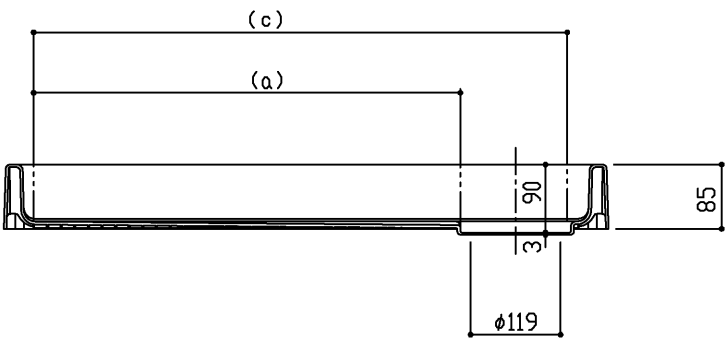
断面A-A
